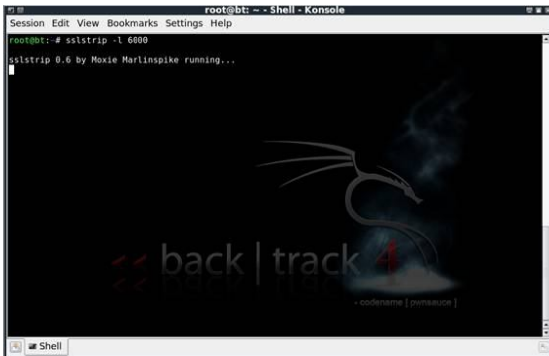
شکل ۲۹. بکارگیری SSLStrip
